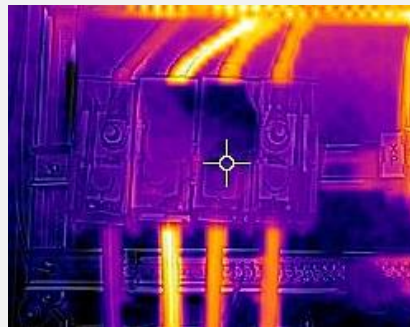
Imagerie Thermique Installation électrique
